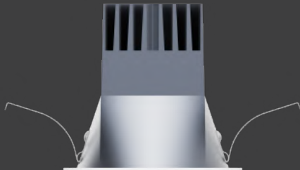
Φ75 Lens: 12W Reflector Cup: 18W
